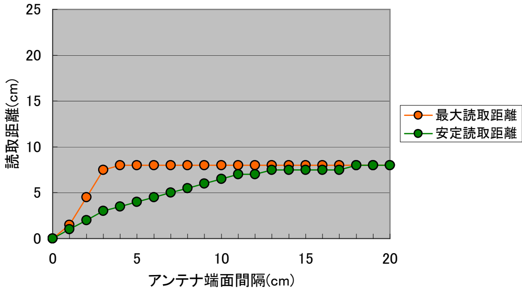
相互干渉による影響(TR3-C202+TR3-A401)
